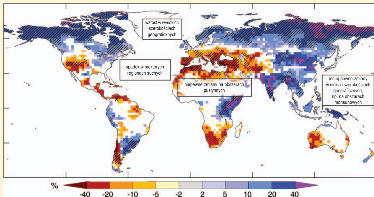
Rysunek 3.5. Wielkoskalowe względne zmiany rocznego odpływu (dostępność wody, w %) dla okresu od 2090 do 2099 w stosunku do lat 1980–1999. Wartości przedstawiają medianę wyników 12 modeli klimatu wykorzystujących scenariusz SRES A1B. Białe kolory pokazują obszary, na których mniej niż 66% z 12 modeli było zgodnych co do znaku zmiany, natomiast dla obszarów zakresowanych, powyżej 90% modeli było zgodnych co do znaku zmiany. Podstawą wyboru 12 modeli była jakość symulacji obserwowanego w XX wieku wielkoskalowego odpływu. Powyższa mapa przedstawia ogólny, wielkoskalowy zarys zmian odpływu i nie odzwierciedla zmian w mniejszych skalach czasowych i przestrzennych. Na obszarach, na których wielkość opadów i odpływu jest bardzo mała (np. pustynie), nawet niewielkie bezwzględne zmiany wielkości odpływu mogą prowadzić do znacznych zmian procentowych. W niektórych regionach znak prognozowanej zmiany odpływu różni się od obecnie obserwowanych trendów. Na niektórych obszarach o przewidywanym wzroście wielkości odpływu mogą zachodzić odmienne zmiany w skali sezonów, takie jak wzrost odpływu w porze wilgotnej i jego spadek z porze suchej. Badania przeprowadzone z wykorzystaniem wyników tylko kilku modeli klimatu mogą znacząco różnić się od zaprezentowanych wyników [WGII rys. 3.4, dopasowany do założeń rys. SYR 3.3; WGII 3.3.1, 3.4.1, 3.5.1].
