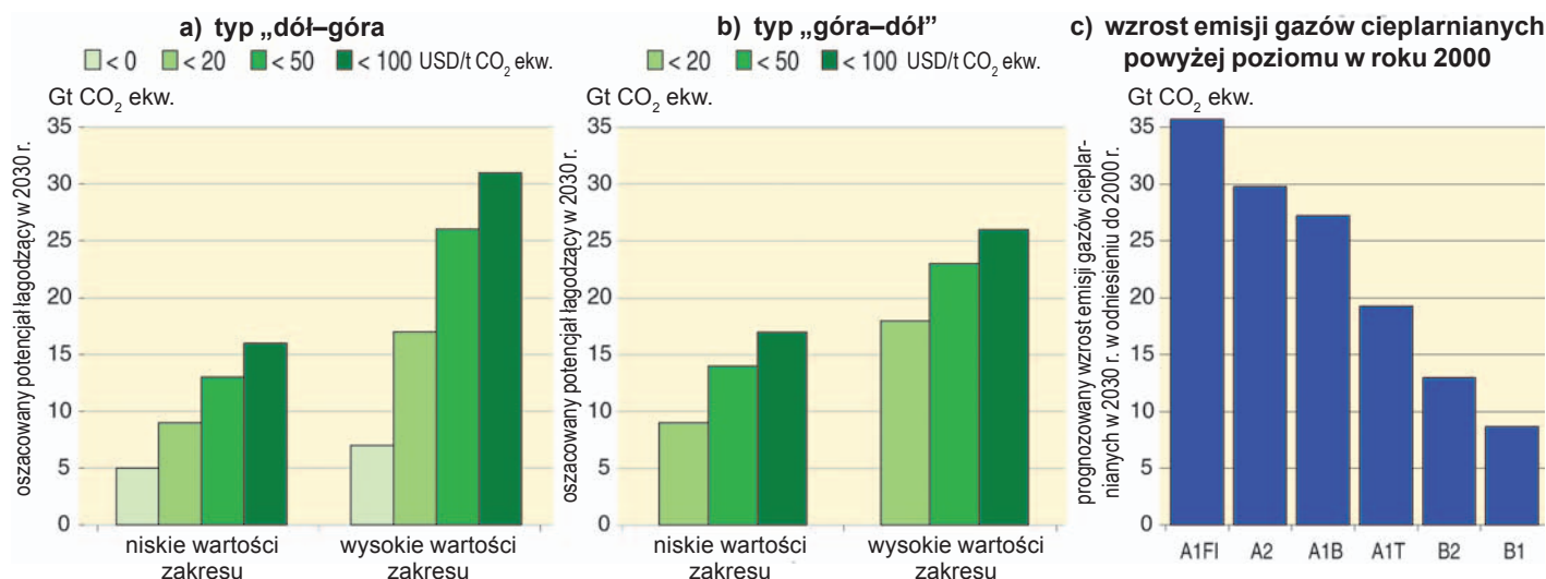
Rysunek 4.1. Globalny ekonomiczny potencjał w 2030 roku oszacowany według analizy typu „dół-góra” (wykres a) oraz typu „góraż-dół” (wykres b) w porównaniu z prognozowanym wzrostem emisji według scenariuszy SRES w odniesieniu do emisji w roku 2000 w wielkości 40,8 Gt CO 2 ekw. (wykres c). Uwaga: Emisja gazów cieplarnianych w 2000 roku nie obejmuje emisji z rozkładu nadziemnej biomasy pozostającej po wyрубie i wylesianiu, jak również z odwadniania gleb torfowych w celu zapewnienia spójności z wynikami scenariuszy SRES {WGIII rys. SPM.4, SPM.5a, SPM.5b}
